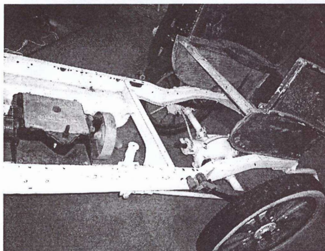
Gearkasse, mellomaksel og kardang. Her har utviklingen "stått stille" i 100 år Denne franske modellen er fra 1905. Snakk om patent som har tålt tidens tann!
